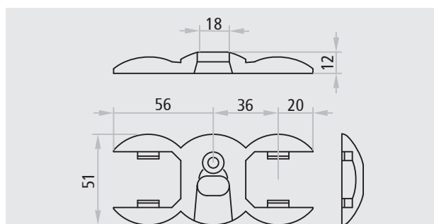
Gâche de sol vantail passif REVER
