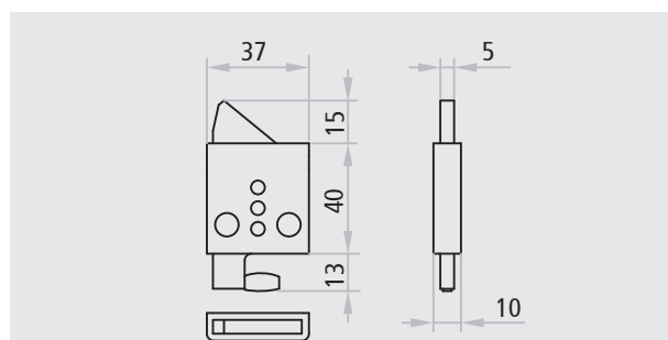
Dispositif haut pour vantail passif PROGET et autres multiusage
