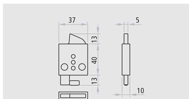
Dispositif haut pour vantail passif UNIVER et REVER
