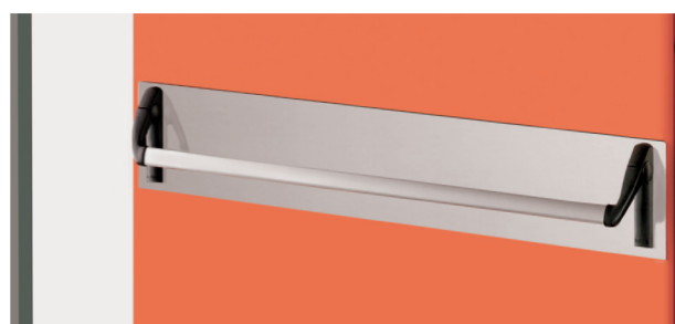
Avec perçages prédisposés pour le passage du carré poignée et du cylindre
