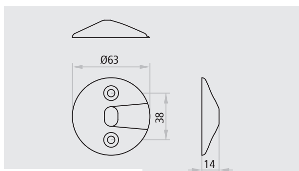
Gâche de sol vantail passif UNIVER
