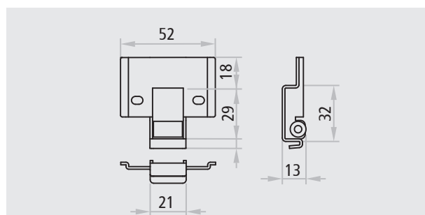
Gâche haute vantail passif PROGET et autres multiusage
