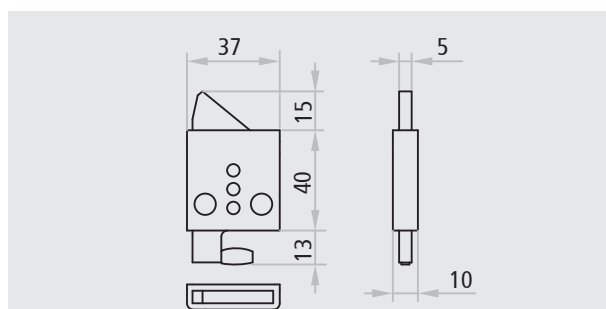
Dispositif haut pour vantail passif PROGET et autres multiusage
