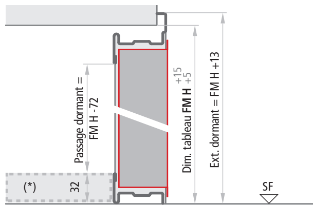
Porte avec battue inférieure interne Coupe verticale
