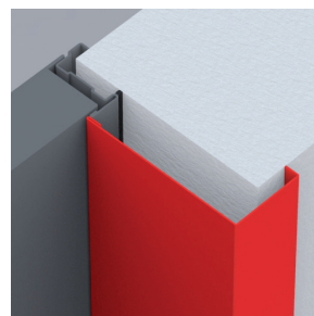
Habillage de tableau IM 11
