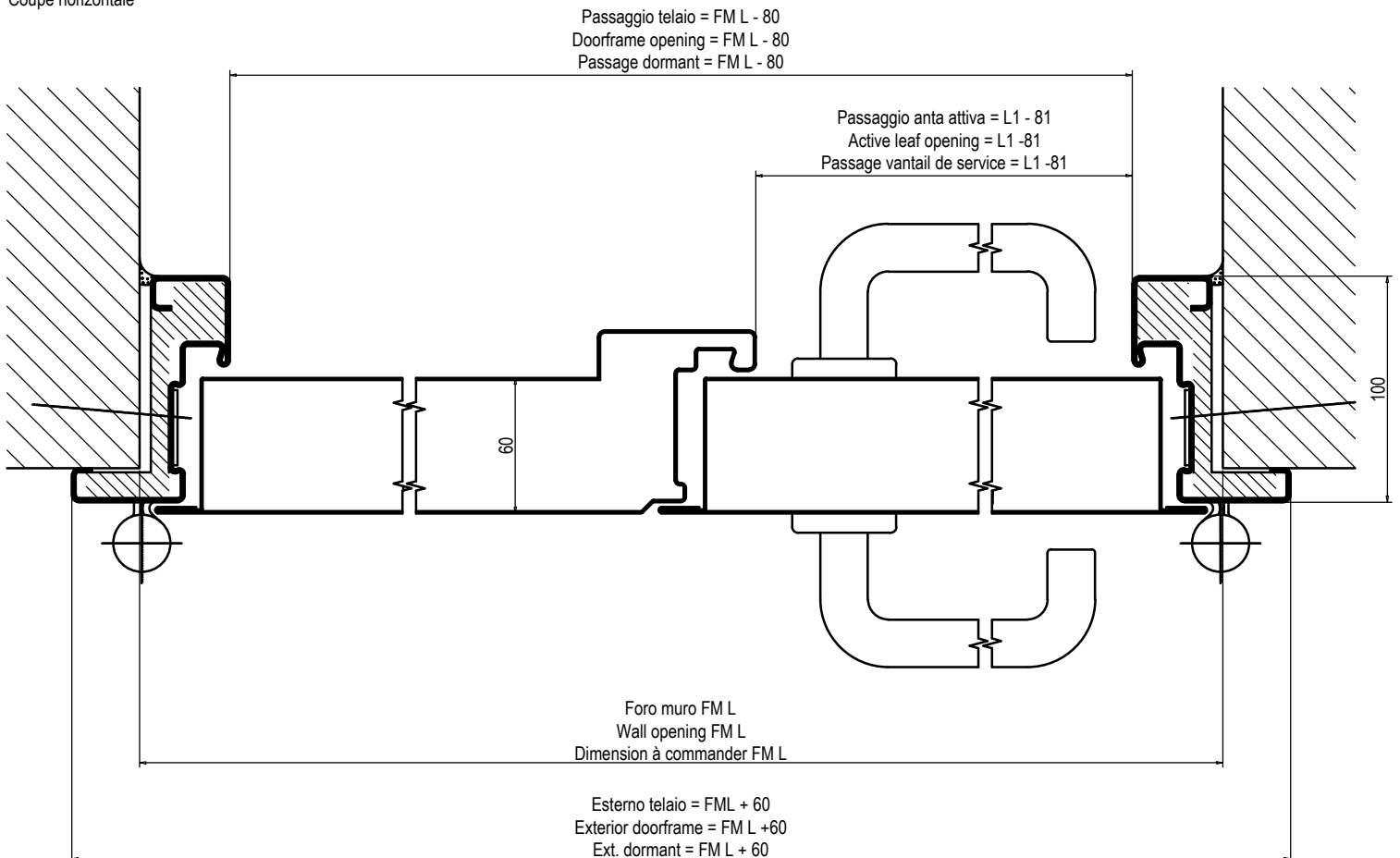
Sezione orizzontale Horizontal cross section Coupe horizontale
