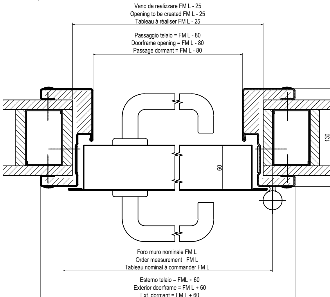
Sezione orizzontale Horizontal cross section Coupe horizontale
