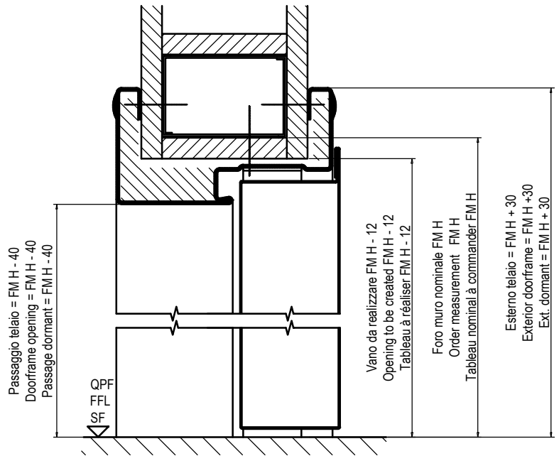
Sezione verticale Vertical cross section Coupe vertical
