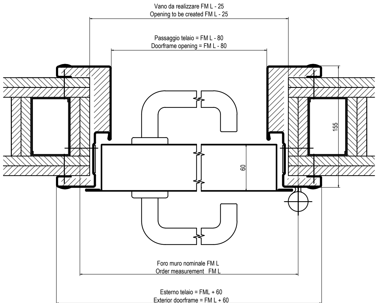
Sezione orizzontale Horizontal cross section
