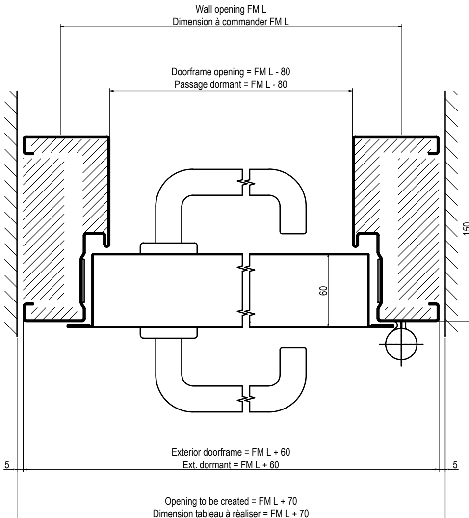
Horizontal cross section Coupe horizontale
