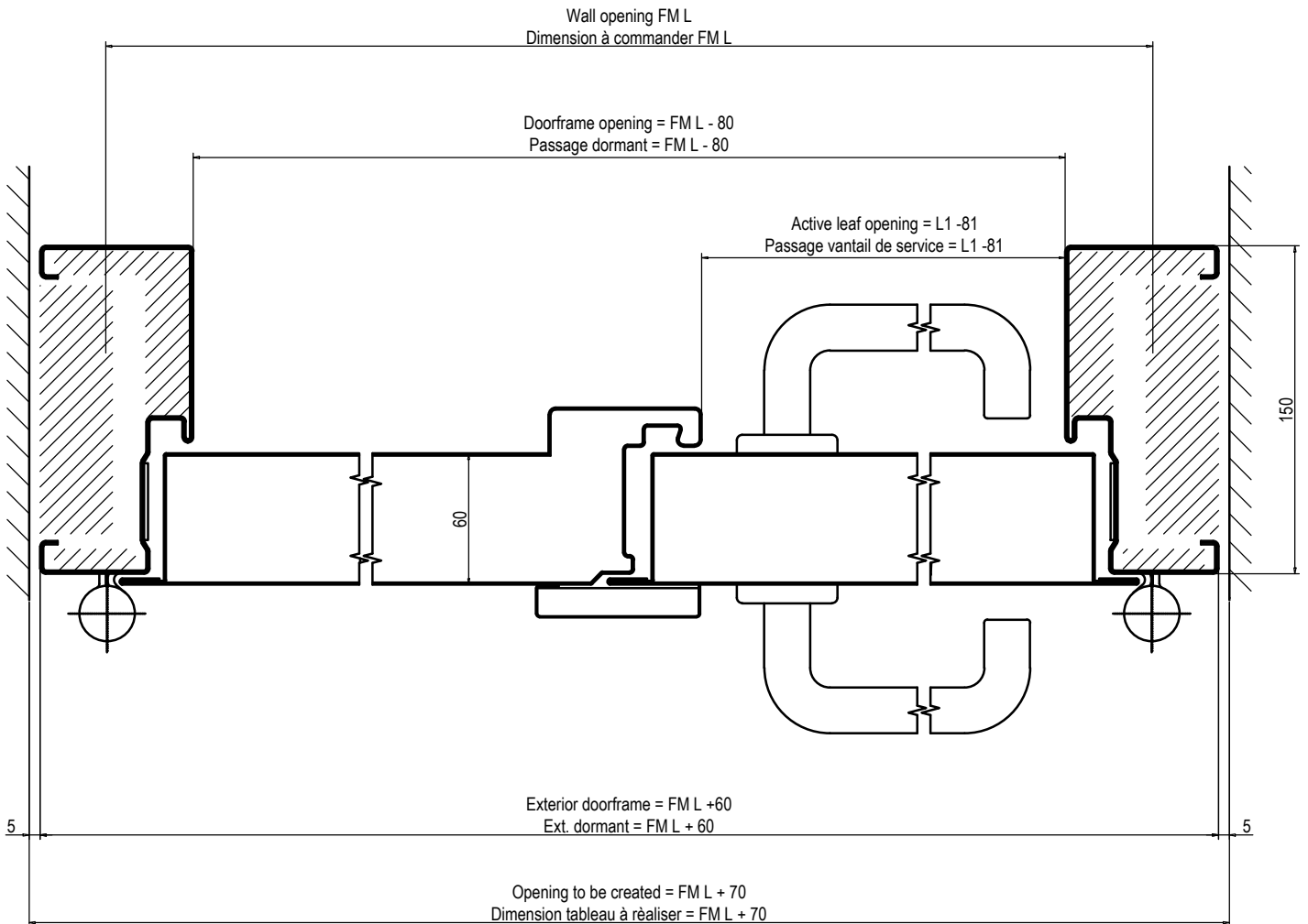
Horizontal cross section Coupe horizontale
