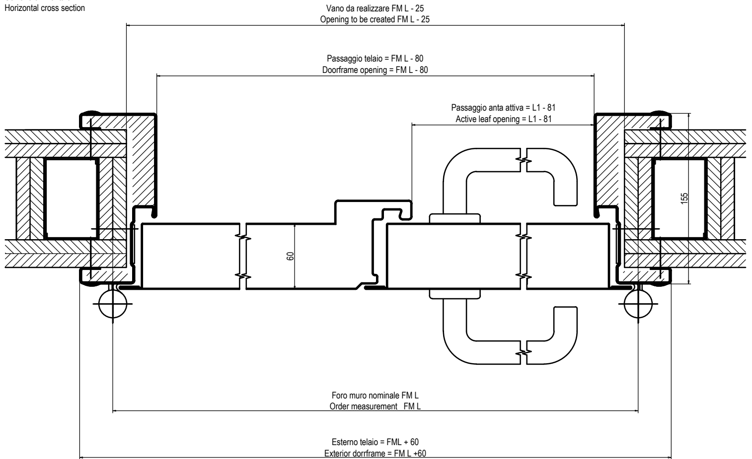
Sezione orizzontale Horizontal cross section
