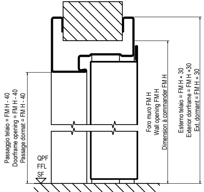
Sezione verticale Vertical cross section Coupe vertical
