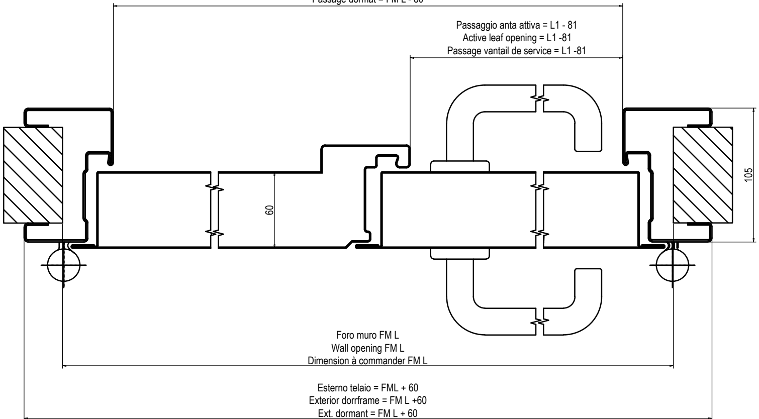
Sezione orizzontale Horizontal cross section Coupe horizontale
