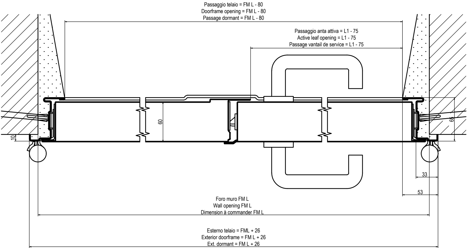
Sezione orizzontale Horizontal cross section Coupe horizontale
