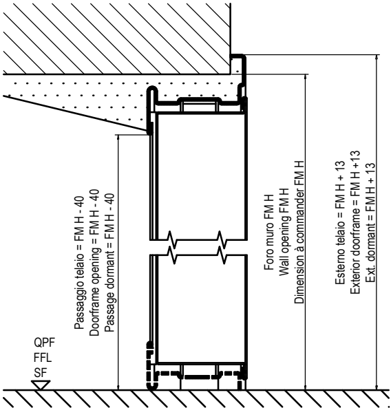
Sezione verticale Vertical cross section Coupe vertical
