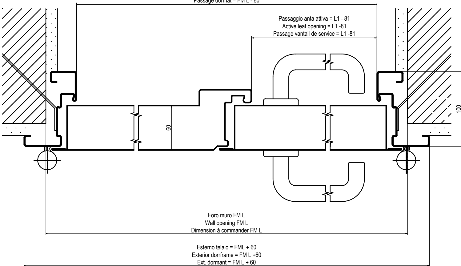
Sezione orizzontale Horizontal cross section Coupe horizontale
