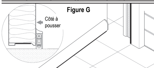
Figure F VERSION AVEC PLINTHES AUTOMATIQUES (Combi Est/GS; Combi Est/GSV, Combi CE Ext/SF, Combi CE Ext/GSV, Combi CE Ext/GS; Combi CE Ext/GSV) Installez la plinthe automatique sur la porte côté poussant en suivant attentivement la fiche des instructions de pose IF01 livrée avec les Combi (voir Figure G). À la fin de l'installation, vérifiez que le joint de la plinthe automatique ne crée pas un obstacle à l'ouverture de la porte. Sinon réglez la plinthe et le joint en suivant la fiche des instructions de pose IF01.
